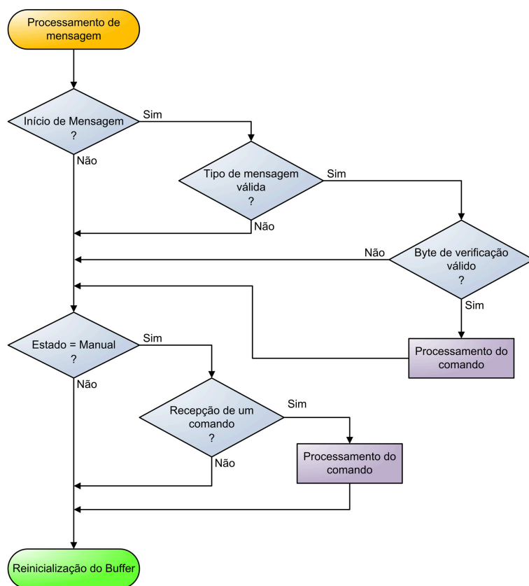
Figura 3.27: Fluxograma da rotina de Processamento de mensagens.
